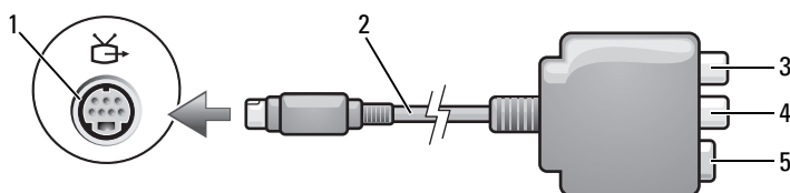
1 S-video TV-out-stik
