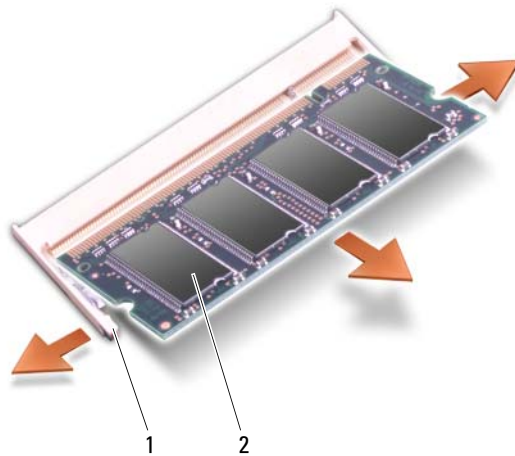
1 fastgørelsesklemmer (2) 2 Hukommelsesmodul
